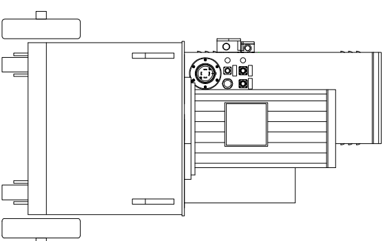
背面図
