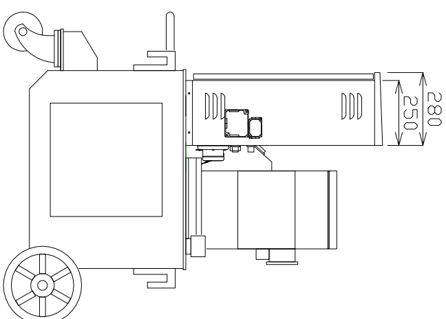
右側面図
